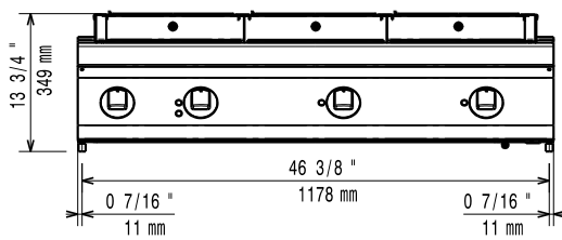
Alzado
